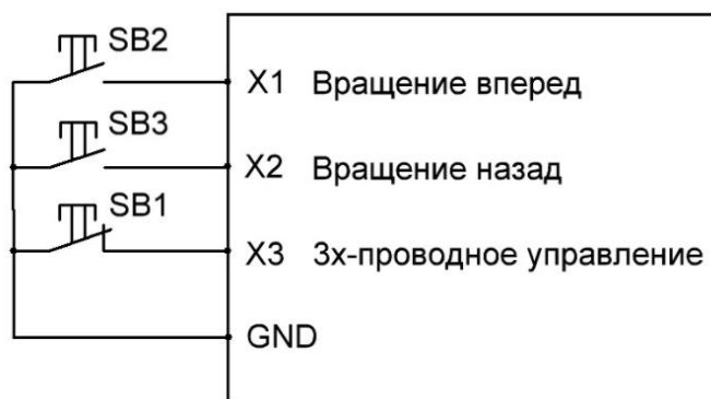
Рис. 5-12 Принципиальная схема трехпроводного режима работы
