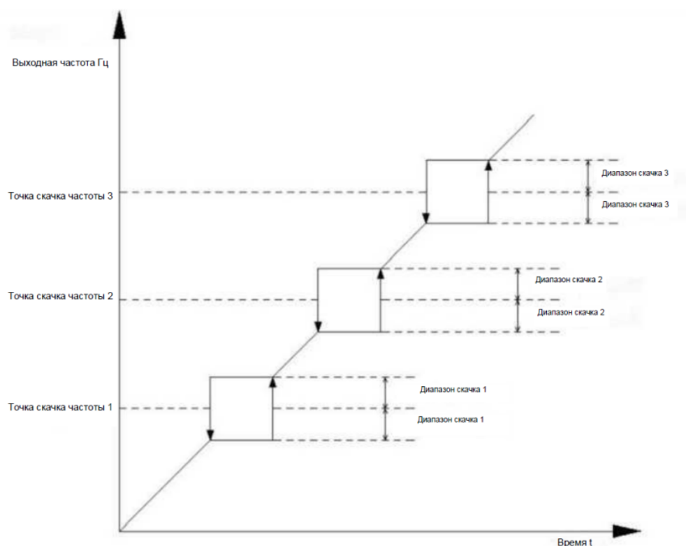
Рис. 5-1 Принципиальная схема переключения частот
