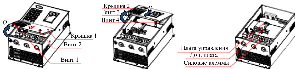
Рис.2-9 ITD...B3 (30~250 кВт)
