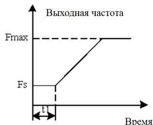
Рис.6-3 Пусковая частота и время выдержки пусковой частоты
