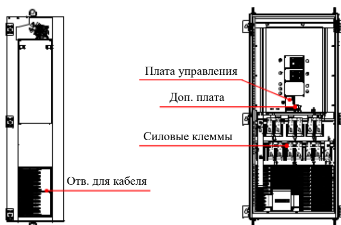
Рис.2-11 ITD...B3 (355~500 кВт)
