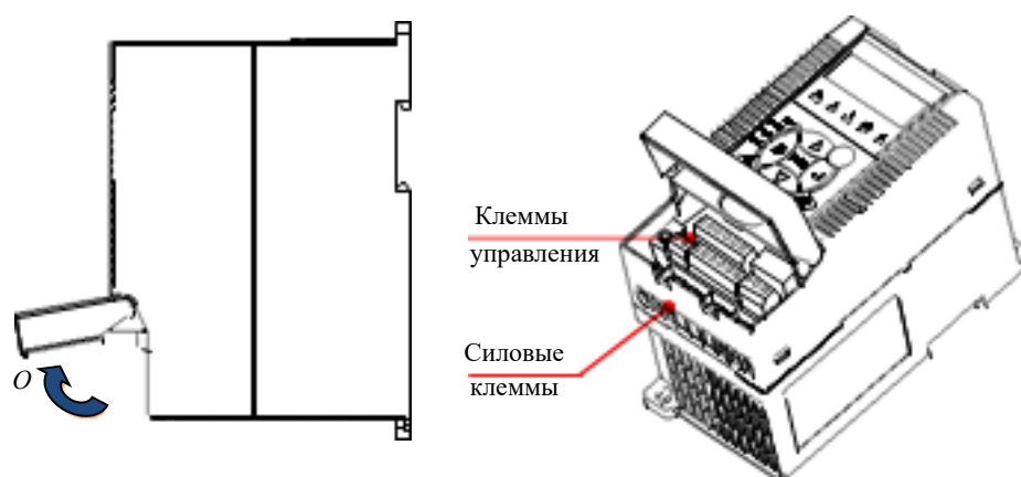
Рис.2-3 ITD...B2 (0.25~1.5 кВт)
