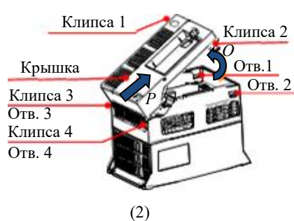
Рис.2-8 (а) ITD...B3 (1.5~11кВт)
