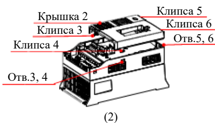
Рис.2-8 (б) ITD...B3 (15~22 кВт)
