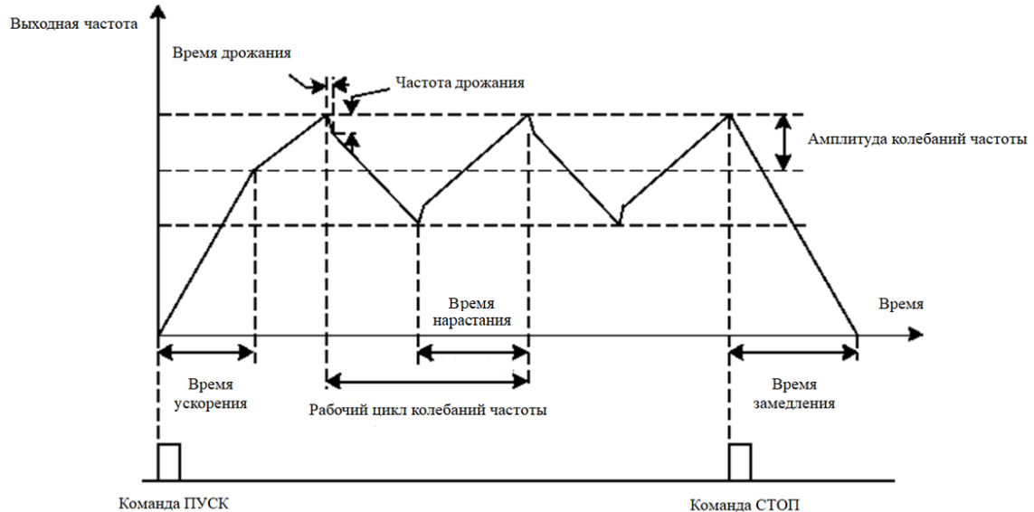
Рис. 6-26 Схема изображения колебаний частоты
