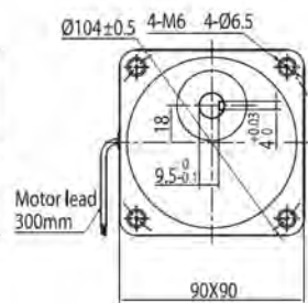
● МОТОР-РЕДУКТОР (Вес: 4,05кг)
